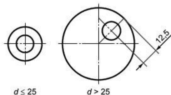
Рисунок 1 - Место вырезки образцов для сортового проката
