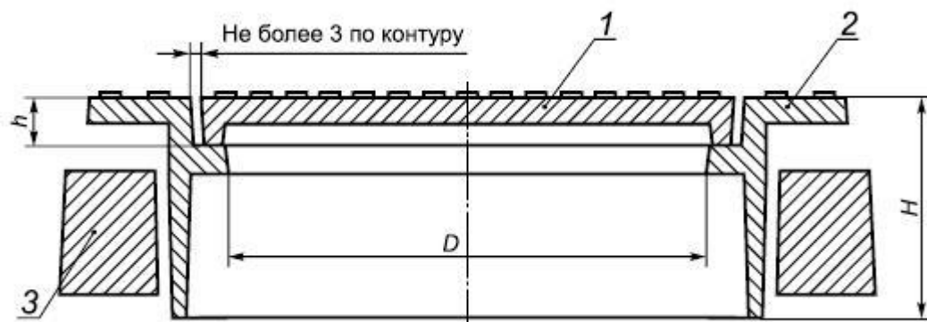
Рисунок А.6 - Люк с крышкой, шарнирно прикрепленной к корпусу
